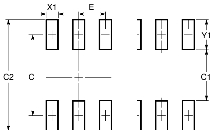
SOT-23, 12L
