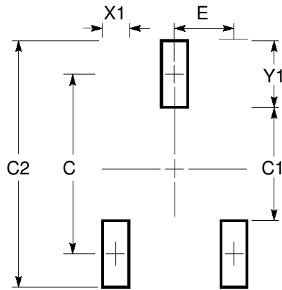
SOT-23, 3L
